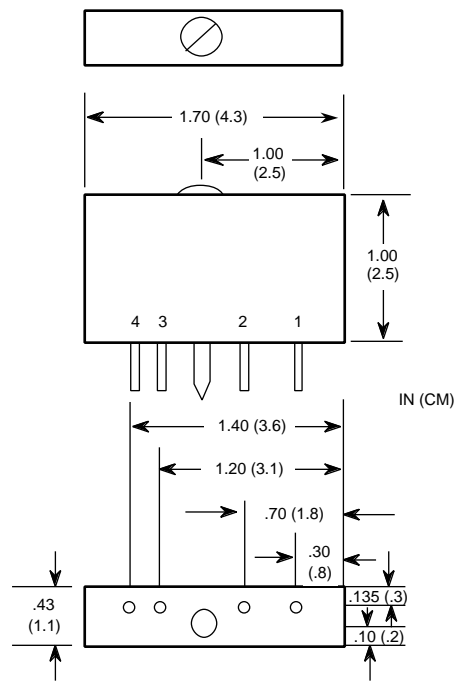
1781-OB5S & 1781-OA5S Slim output modules
