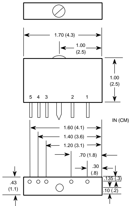
1781-IB5S & 1781-IA5S Slim input modules
